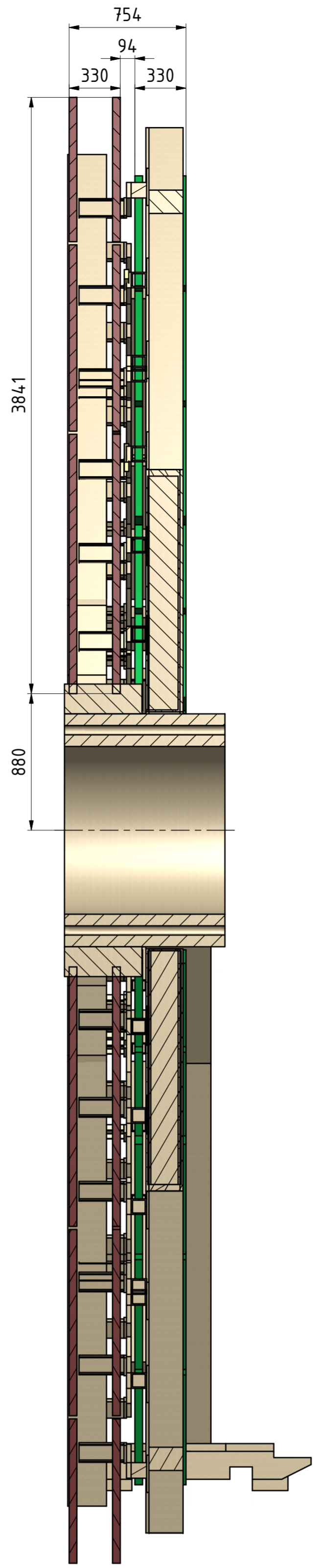
A-A ( 1 : 25 )
