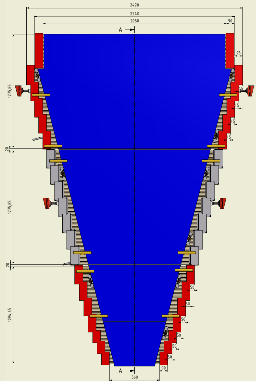
A-A ( 1 : 10 )
