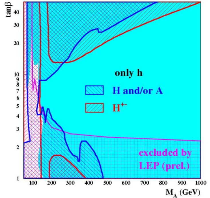
MSSM
