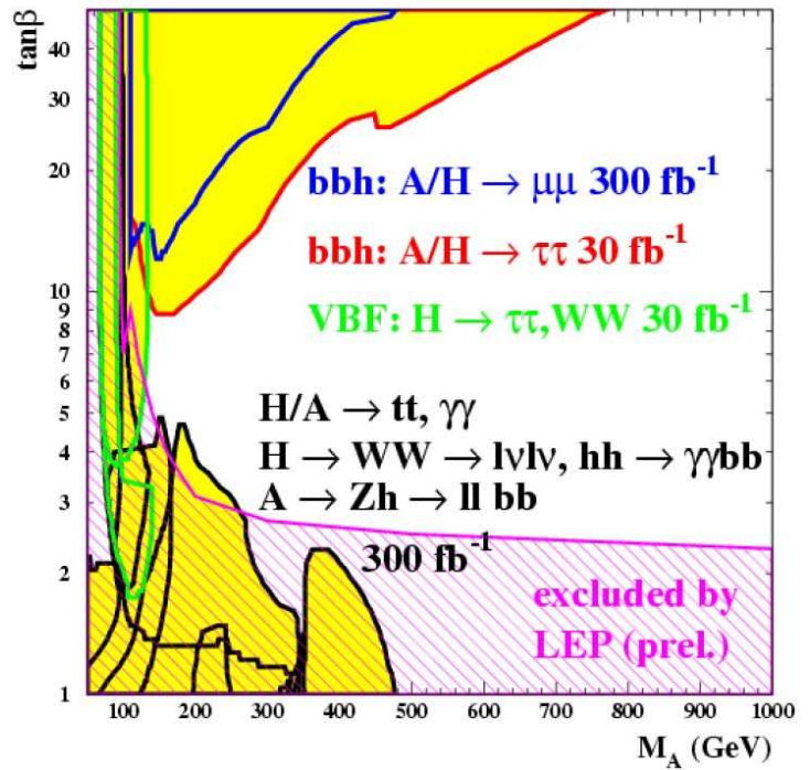
MSSM
