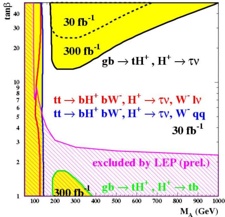
MSSM
