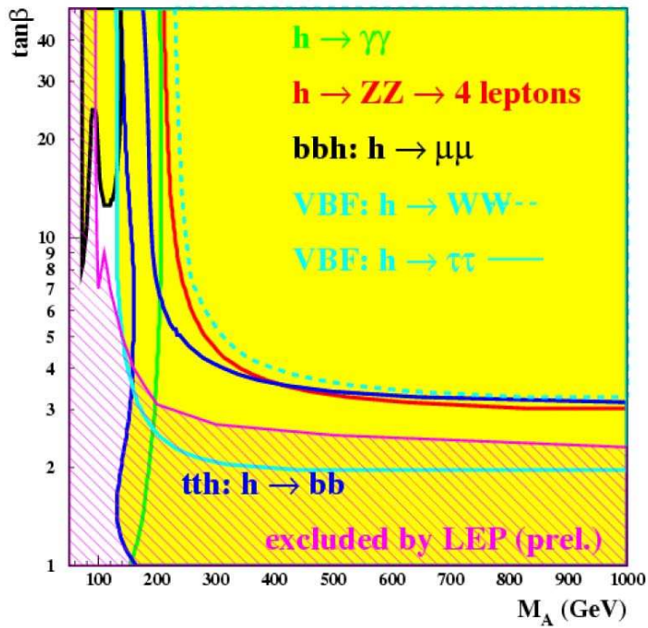
MSSM
