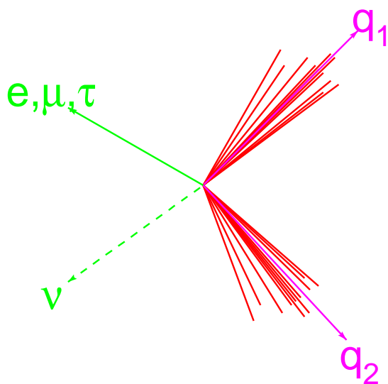
semileptonisch
