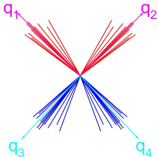
hadronisch
